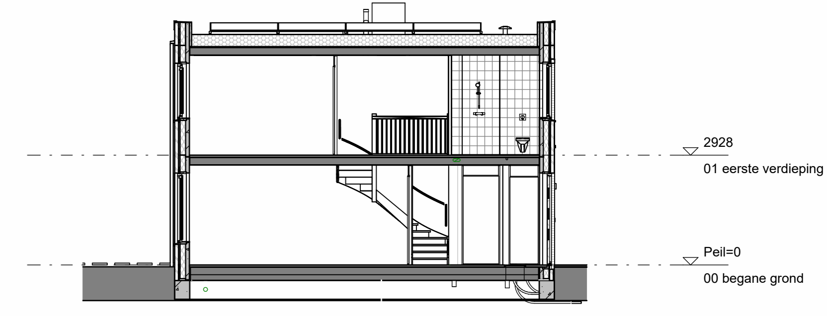
doorsnede D-D
