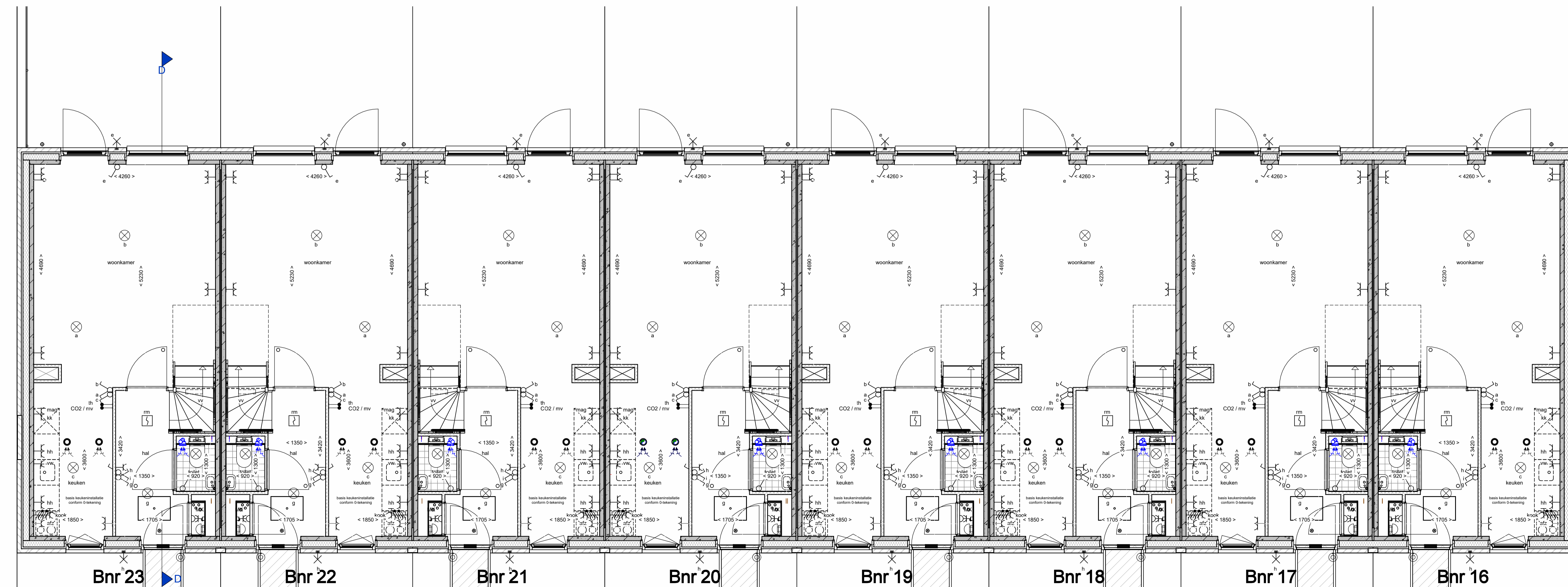
begane grond
