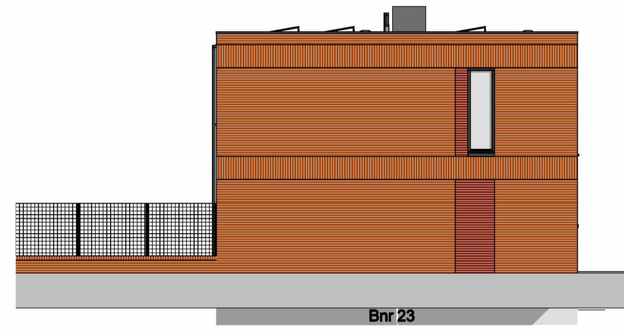
linker zijgevel
