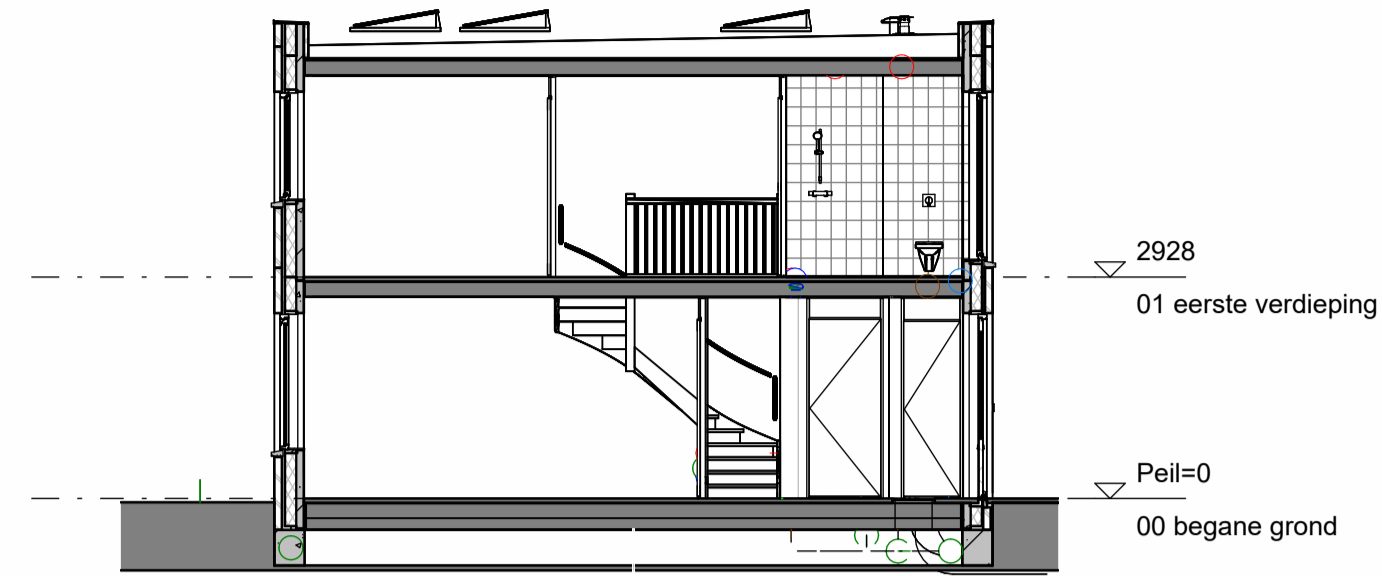
doorsnede D-D
