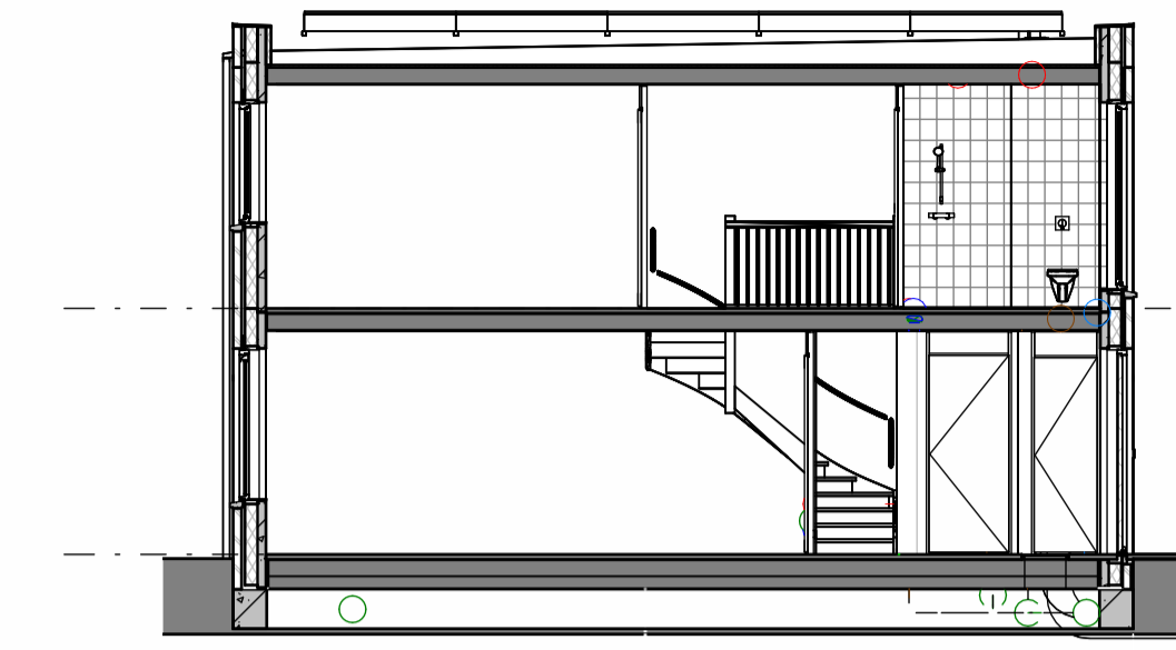
doorsnede A-A
