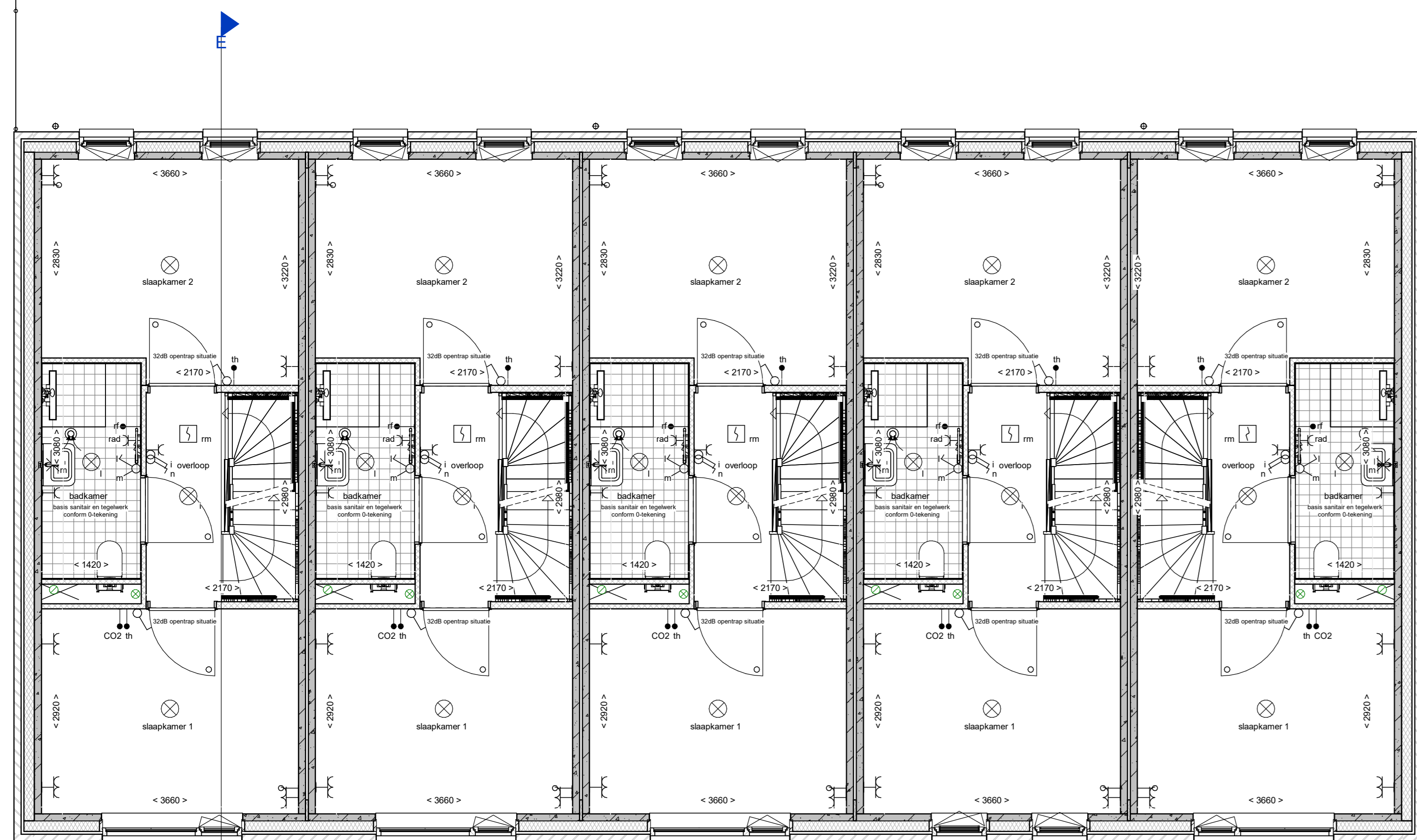
BNR 28 BNR 27 BNR 26 BNR 25 BNR 24 1e verdieping schaal 1 : 50
