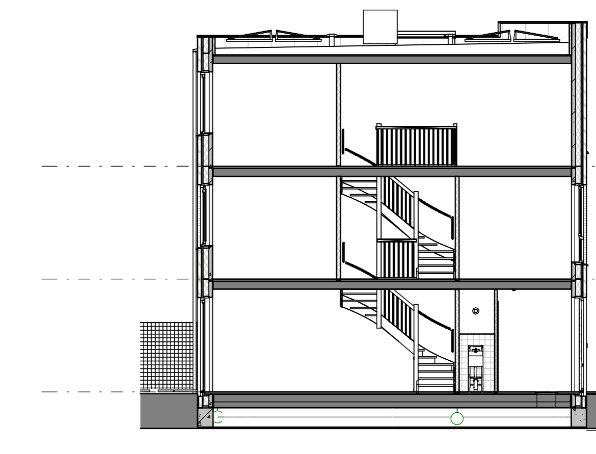
doorsnede E-E schaal 1 : 100
