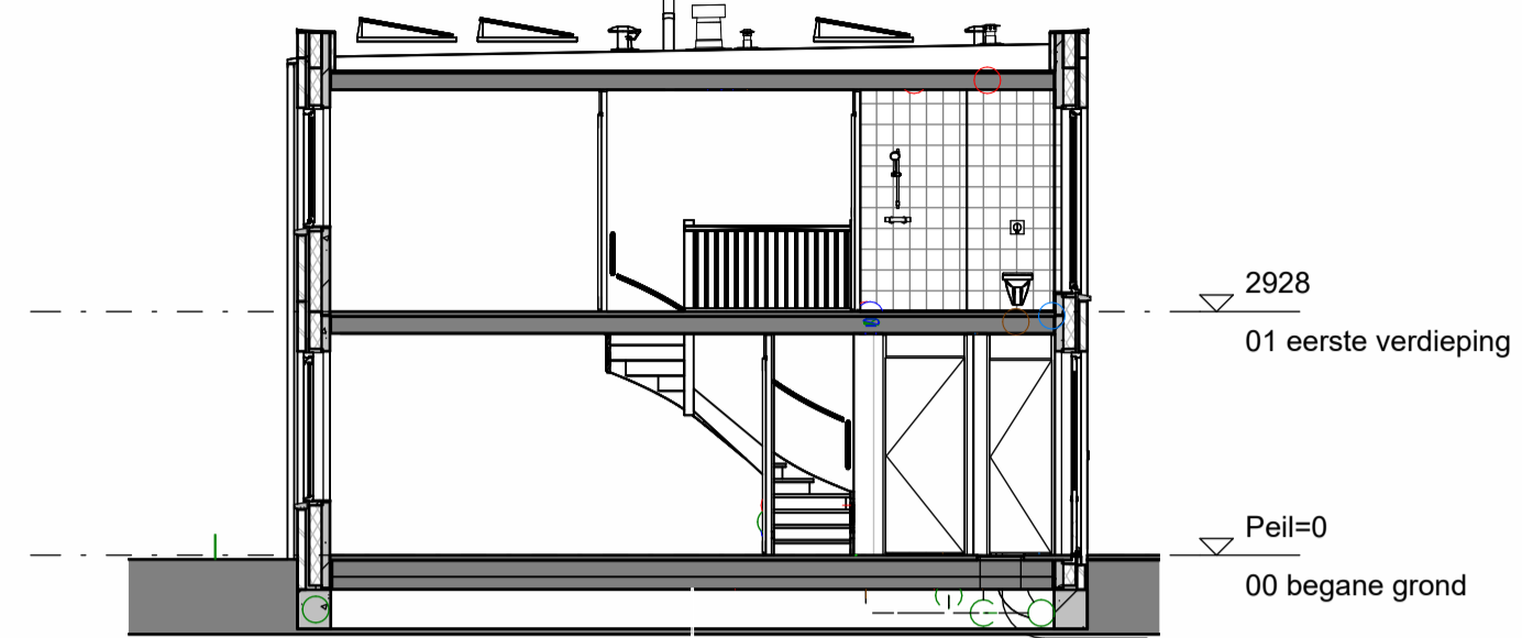
doorsnede G2-G2 schaal 1 : 100
