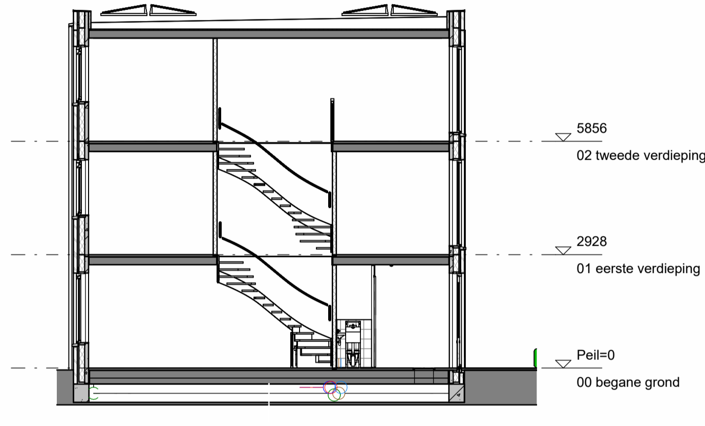
doorsnede G1-G1 schaal 1 : 100
