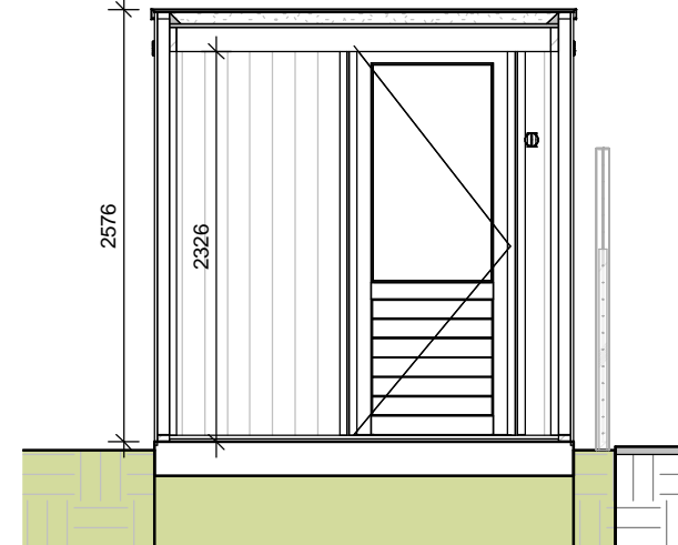
Dubbele berging breed_B
