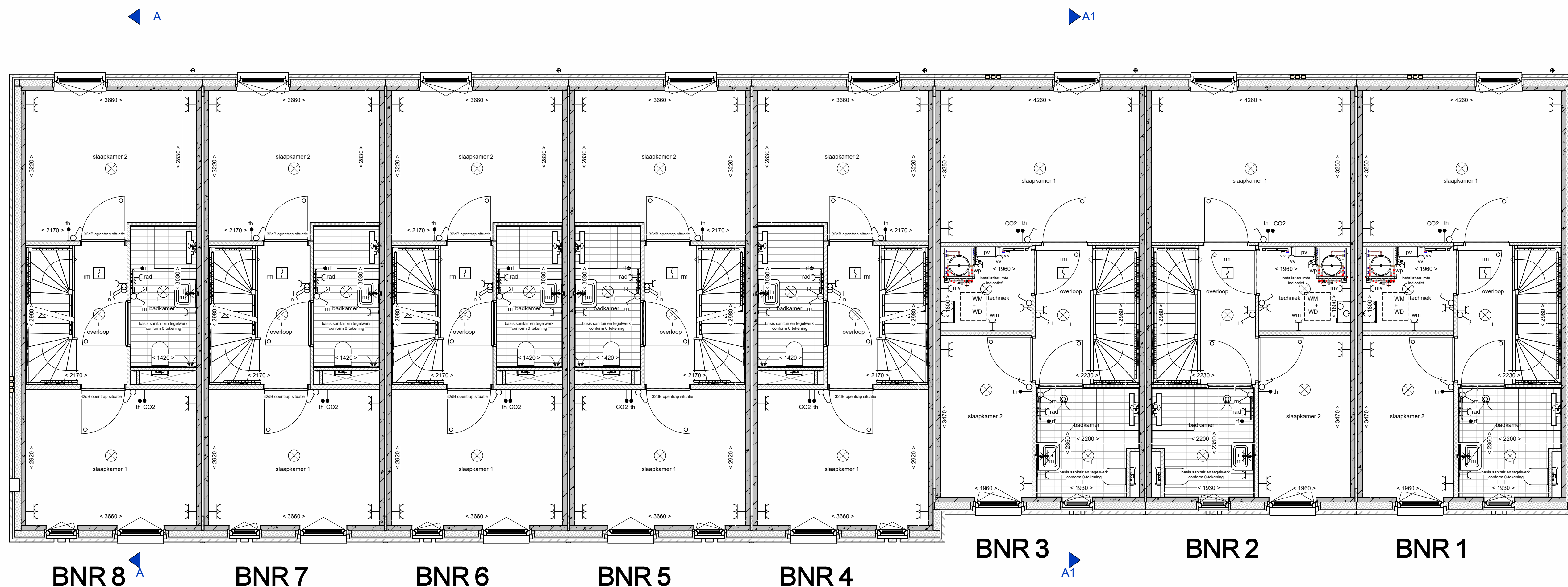
1e verdieping schaal 1 : 50
