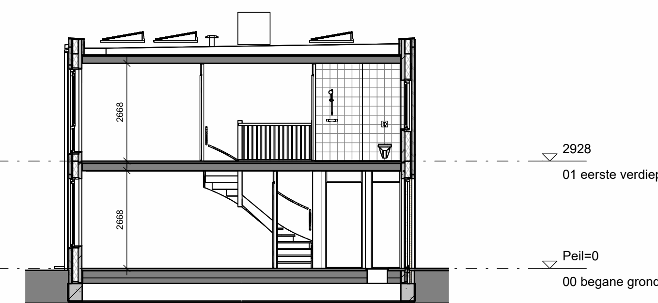
doorsnede A1-A1
