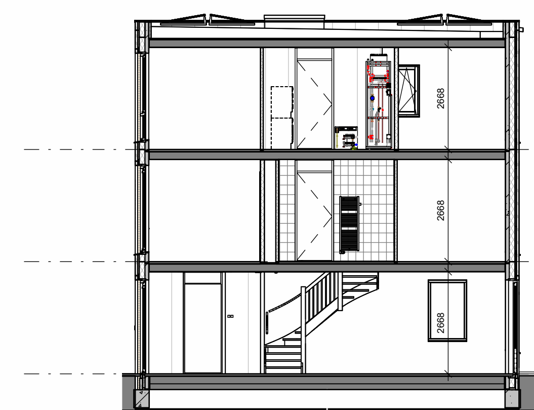
doorsnede A-A
