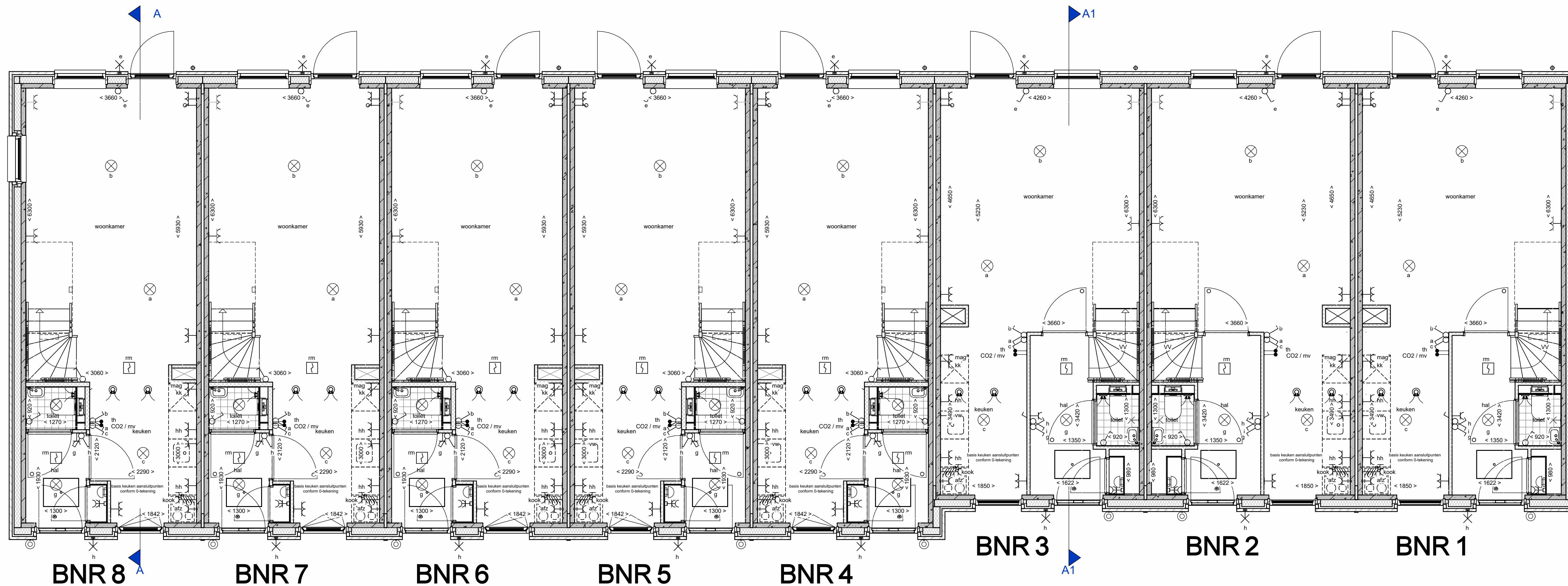
begane grond schaal 1 : 50
